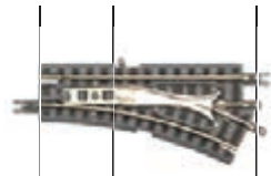
7297023 (R023) Elektr. Weiche rechts, R127-26°, 55 mm, mit 1 x angeschnittenem geraden Gleis, 55 mm (1 Stück)
