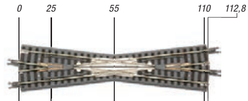
7297020 (R020) Kreuzung 13°, 112,8 mm, mit 2 x Ausgleichsgeleis 53,6 mm (1 Stück)
