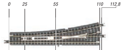
7297039 (R039) Elektr. Weiche links, R490-13°, 110 mm, mit 1 x angeschnittenem geraden Gleis, 110 mm (1 Stück)
